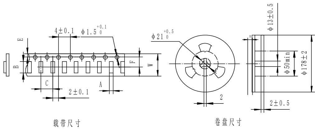
图3 编带尺寸
