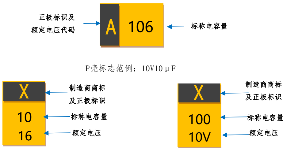
A壳标志范例：16V10 \mu F
